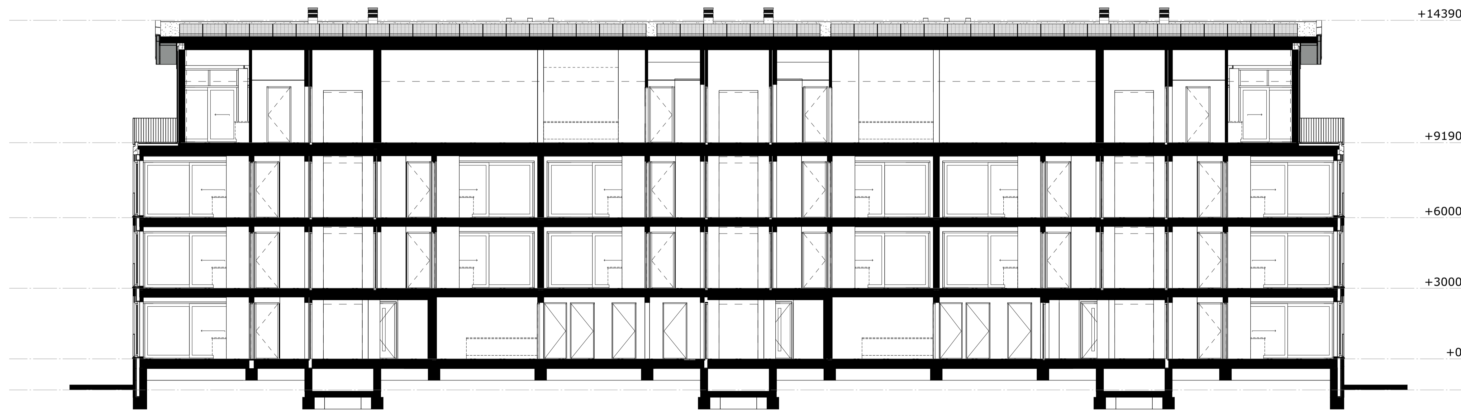
doorsnede D
