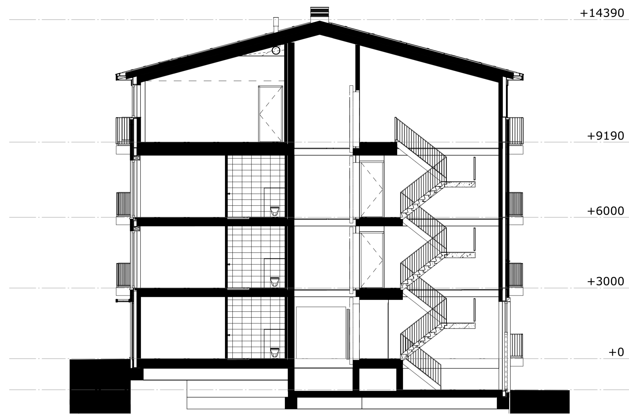
doorsnede A
