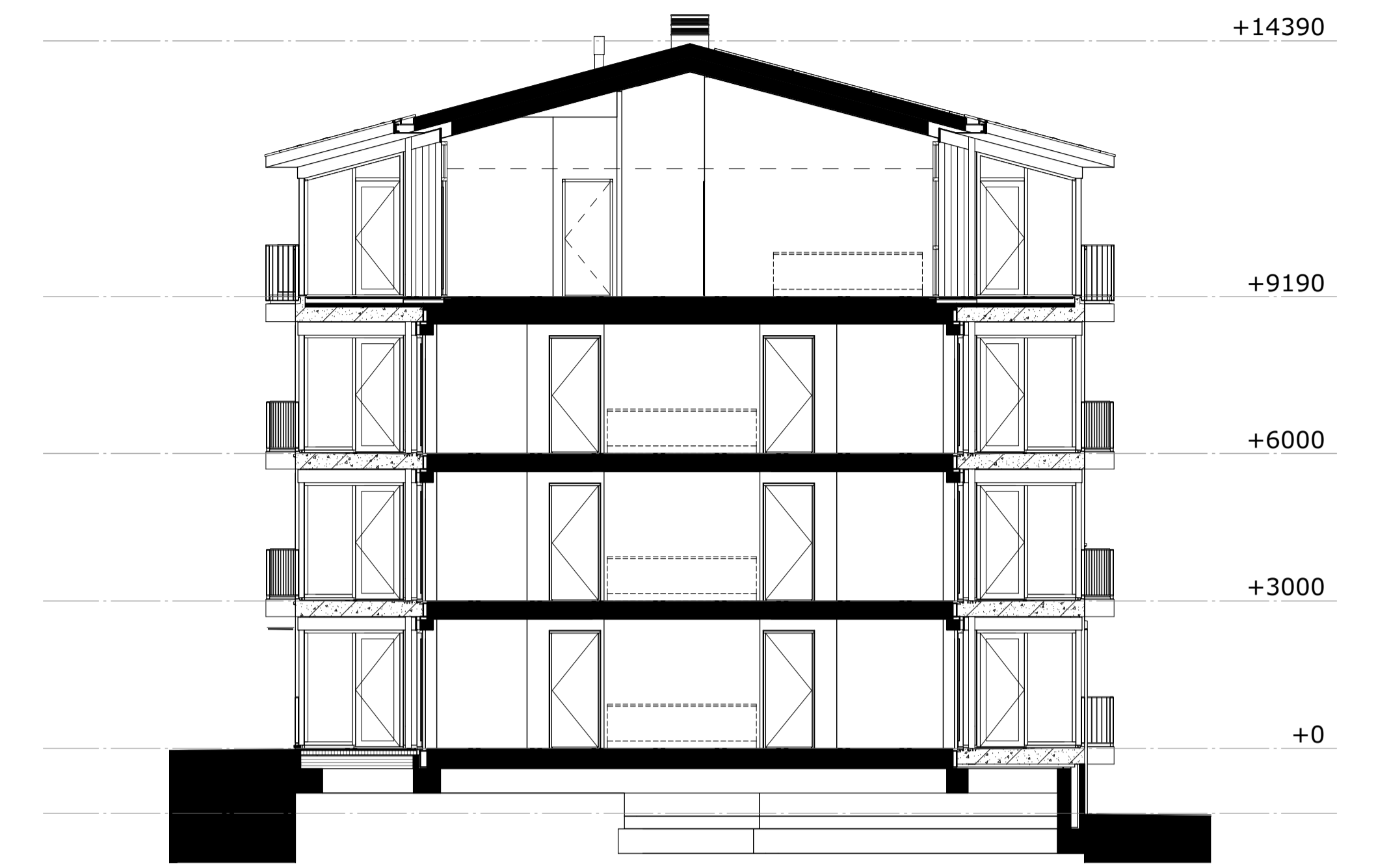
doorsnede C
